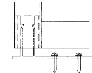
ANCHORS TYPE 'C' JAMB CLIP ANCHORS
