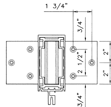
ANCHORS TYPE 'C' JAMB CLIP ANCHORS
