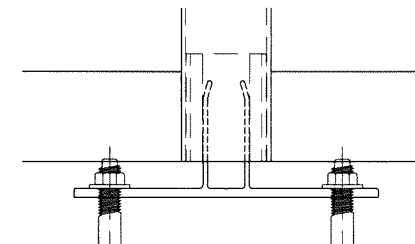
ANCHORS TYPE 'B' MULLION CLIP ANCHORS
