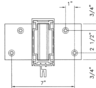
ANCHORS TYPE 'A' & 'B' JAMB CLIP ANCHORS
