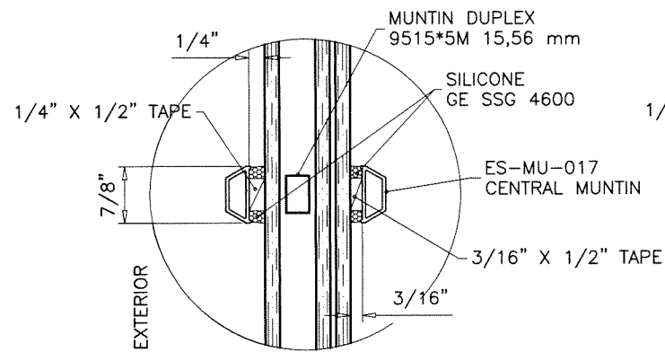
ALUMINUM MUNTINS OPTIONAL
