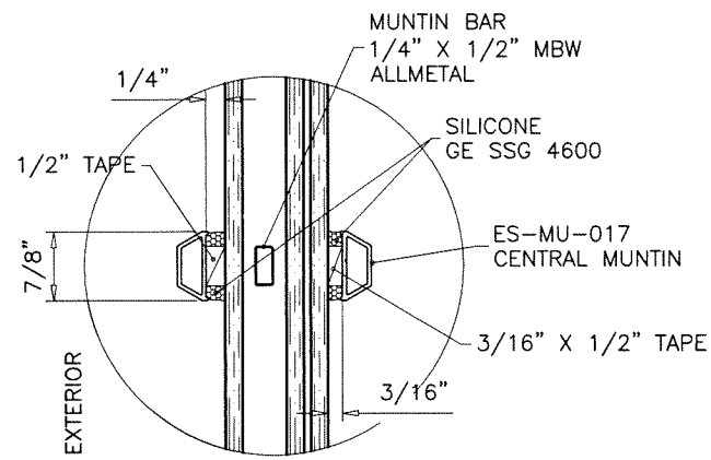
ALUMINUM MUNTINS OPTIONAL
